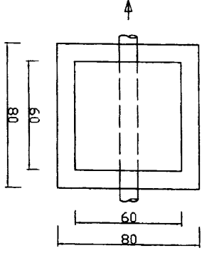
แปลนบ่อแมนโฮล
