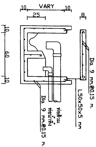
รูปตัด
